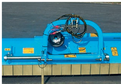
Attacco con spostamento idraulico Linkage with hydraulic offset Enganche con desplazamiento hidráulico
