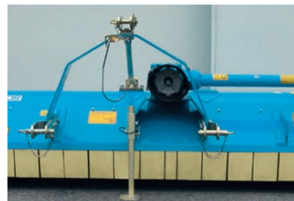
Attacco fisso due posizioni 2-point-fixed linkage Enganche fijo con dos posiciones
