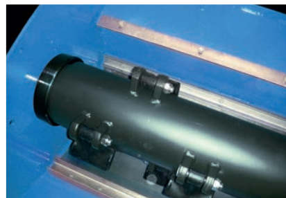
Lamiera di consumo e doppio controcoltello Wear and tear metal sheet and double counterknife Chapa de blindaje y doble contracuchillas
